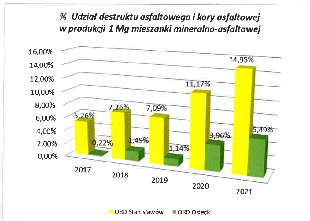
Wykres 11. Udział destruktu asfaltowego w produkcji MMA.
