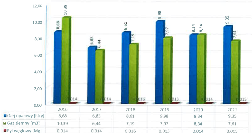
Wykres 10. Wskaźniki zużycia paliwa do produkcji MMA
